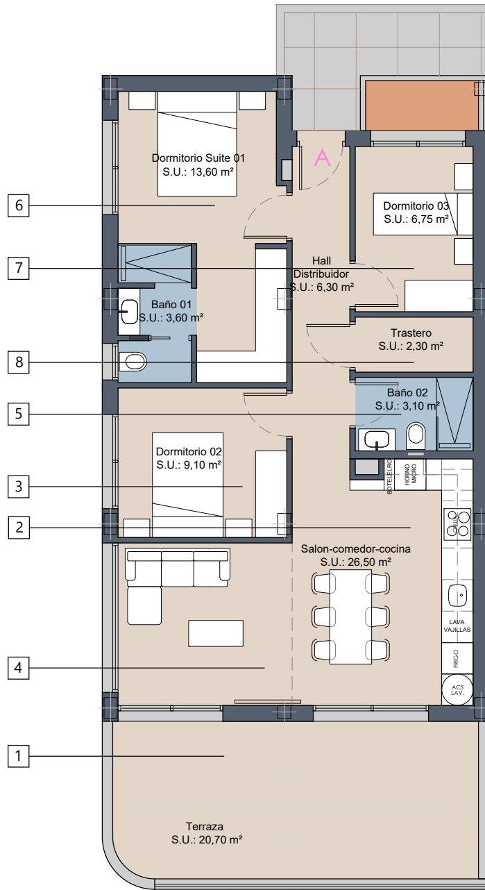
PLANTA PRIMERA
